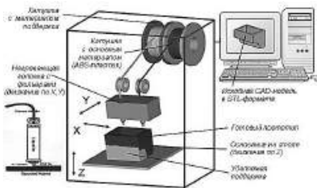
Рис. 1. Принцип создания моделей-прототипов по FDM-технологии
