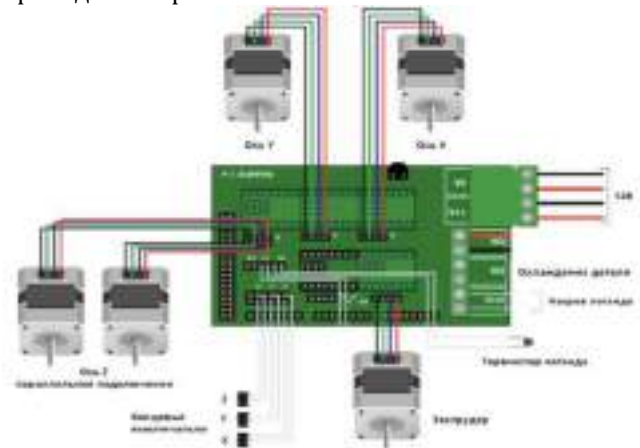
Рис. 3. Схема подключения электроники 3D-принтера
