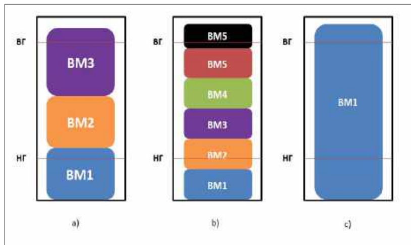
Рисунок 2. Типичные ситуации превышения верхнего порогового значения загрузки процессора (VG — верхняя граница, NG — нижняя граница).
