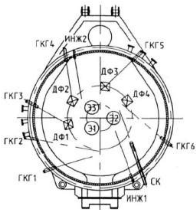
Рис. 5 – Схема расположения горелок и фурм в ДСП-100 НМЗ: ГКГ1 – ГКГ6 – стеновые газокислородные горелки; ИНЖ1, ИНЖ2 – инжекторы для глубокого вдувания карбюризатора; ДФ1 – ДФ4 – донные газо-кислородные фурмы; СК – сверхзвуковое копьё для подачи кислорода и карбюризатора.
