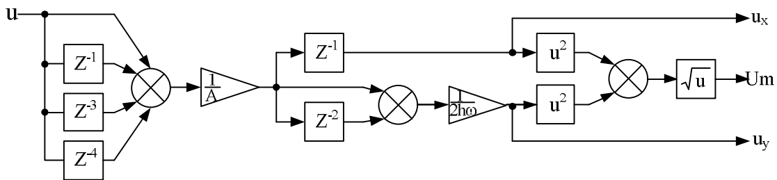
Рисунок 2 – Структурная схема блока определения комплексных значений сигнала
