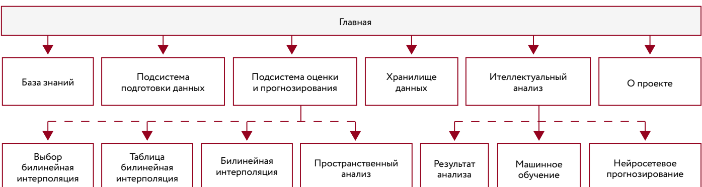
Рис. 4. Схема интеллектуальной информационной системы
