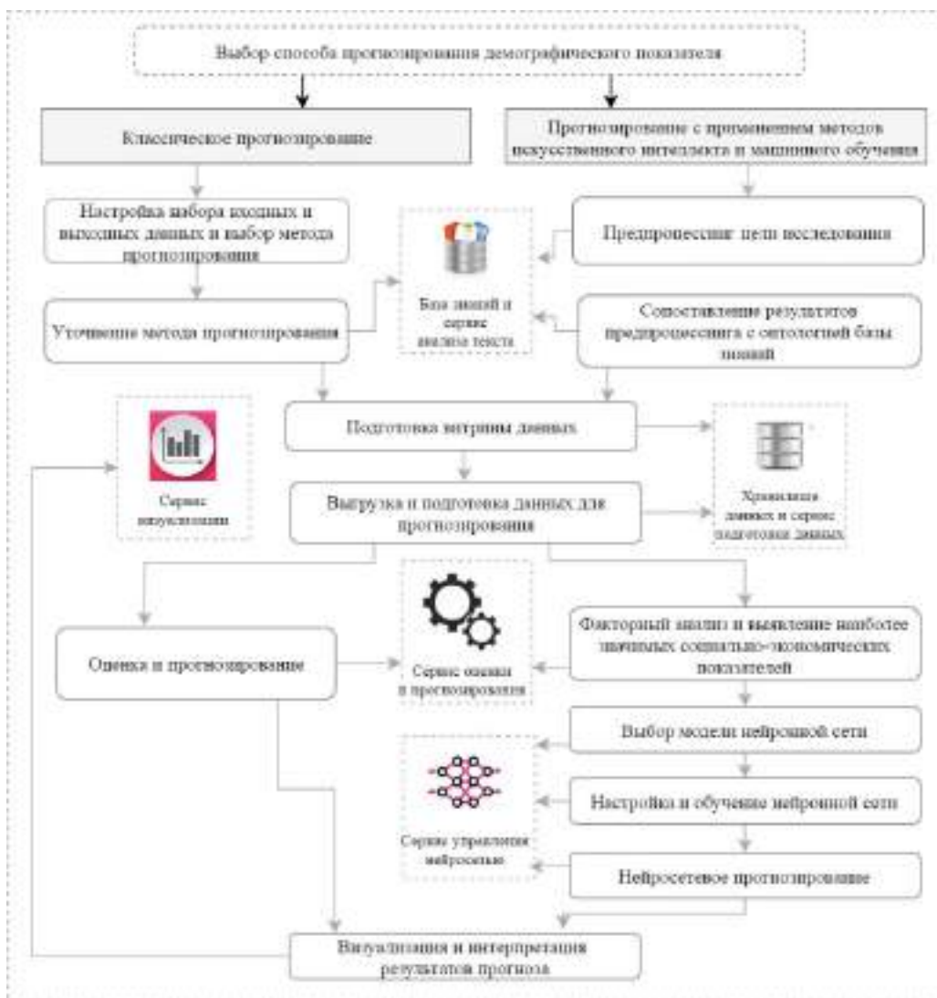
Рис. 2. Обобщенная схема технологических процессов в интеллектуальной информационной системе демографического прогноза региона
