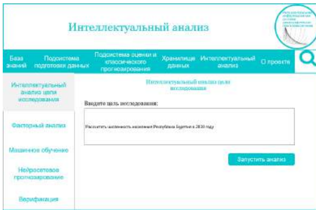
Рис. 13. Прототип интерфейса задания цели исследования на естественном языке
