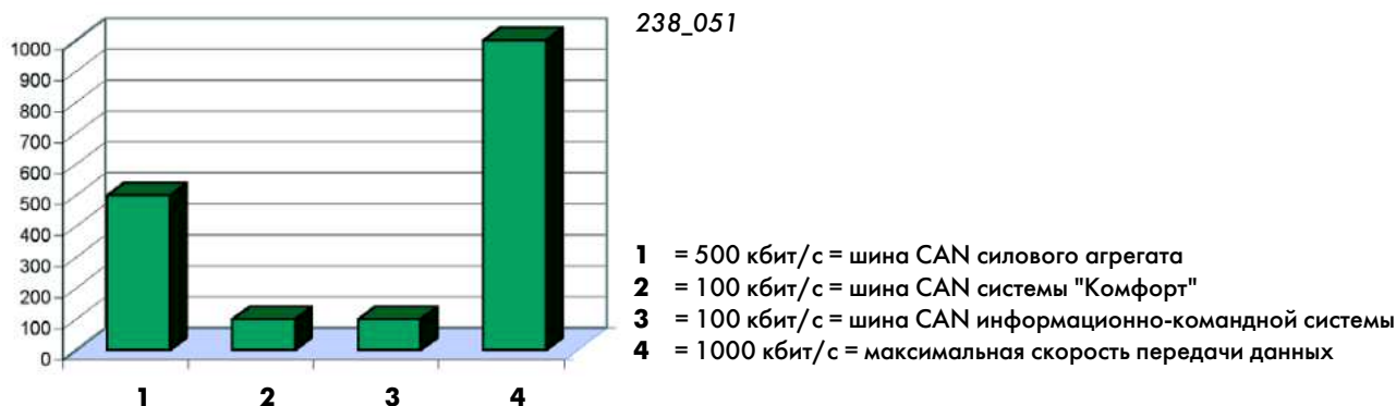
Скорости передачи данных в системе CAN
