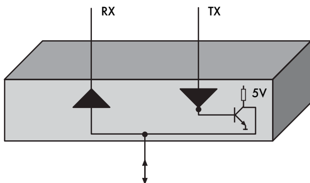
Трансивер с подключенным проводом TX
