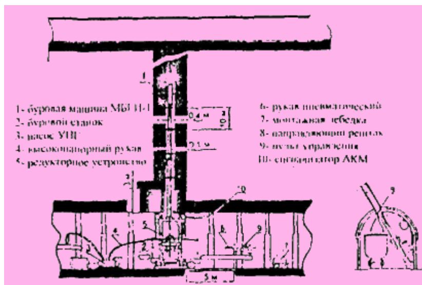
Рисунок 4. Технологическая схема бурения скважин МБГИ-1
