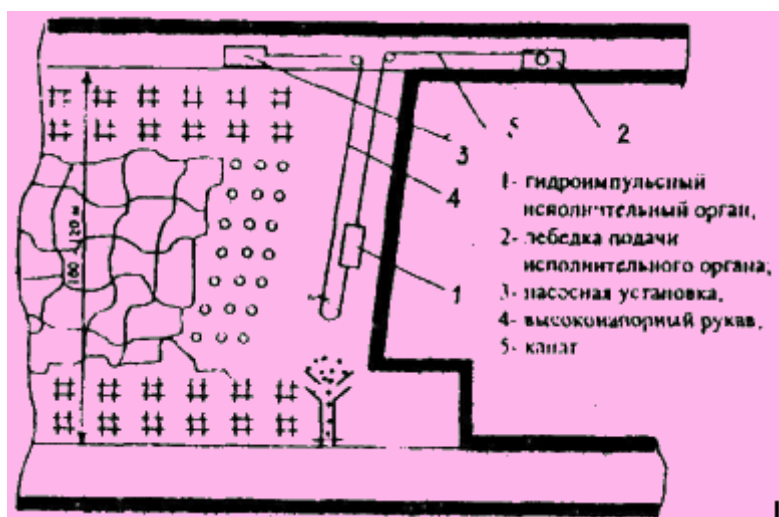
Рисунок 2. Отработанная технологическая схема выемки крутопадающего пласта гидроимпульсной установкой ГИУВм-1
