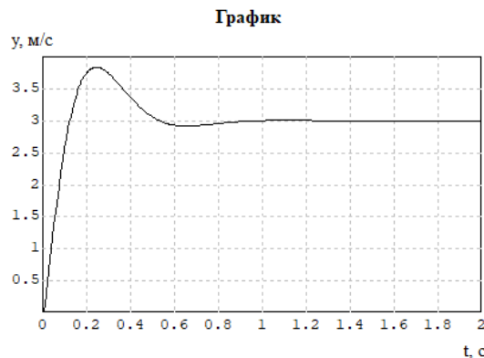
Рисунок 4 - Реакция системы на обработку заданной скорости транспортировки
