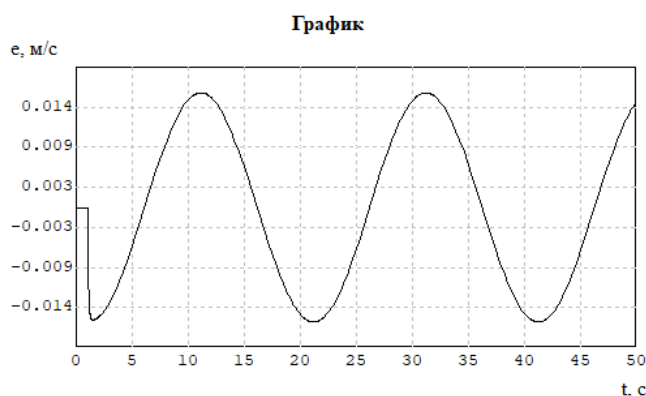
Рисунок 6 - График изменения ошибки e(t) системы ПИ регулятором при гармоническом входном воздействии f(t) = 0,6 \sin 0,314t
