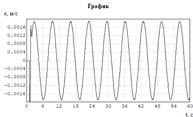
Рисунок 7 - График изменения ошибки e(t) системы с обобщенным регулятором при гармоническом возмущающем воздействии f(t) = 0,6 \sin 0,942t
