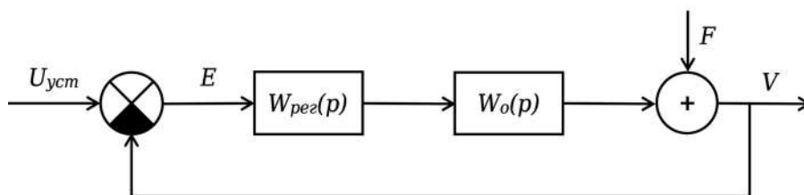
Рисунок 2 - Структурная схема системы
