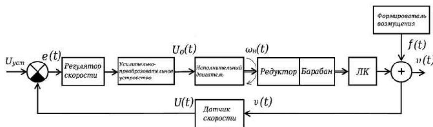
Рисунок 1 - Функциональная схема системы автоматического регулирования скорости ленточного конвейера
