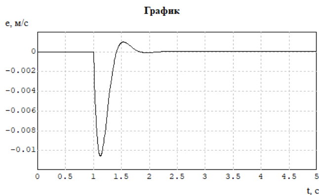
Рисунок 5 - График изменения ошибки e(t) системы с обобщенным регулятором при гармоническом возмущающем воздействии f(t) = 0,6 \sin 0,314t
