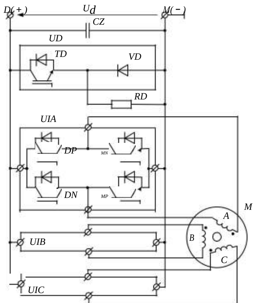
Рис. 1 Схема альтернативного тягового электропривода
