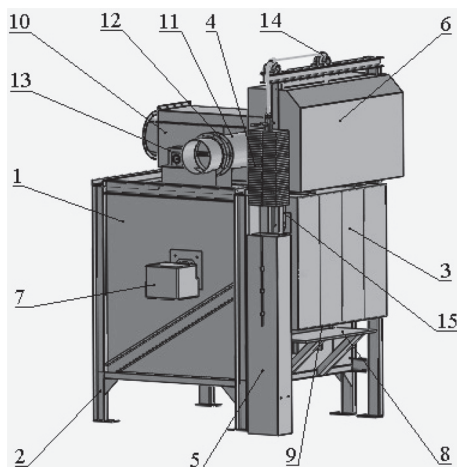
Рис. 1. Общий вид печи
