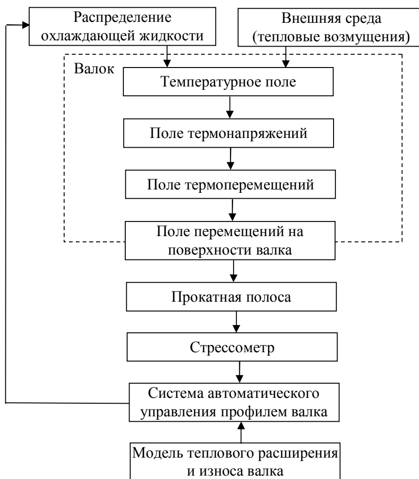
Рисунок 2 – Блок-схема процесса управления профилем вала
