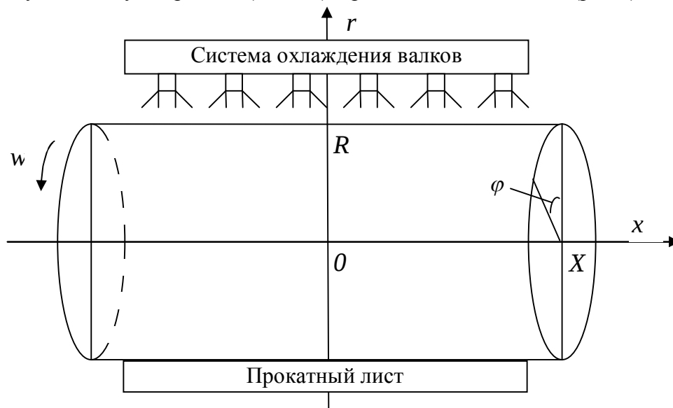
Рисунок 1 – Валок прокатного стана в цилиндрической системе координат
